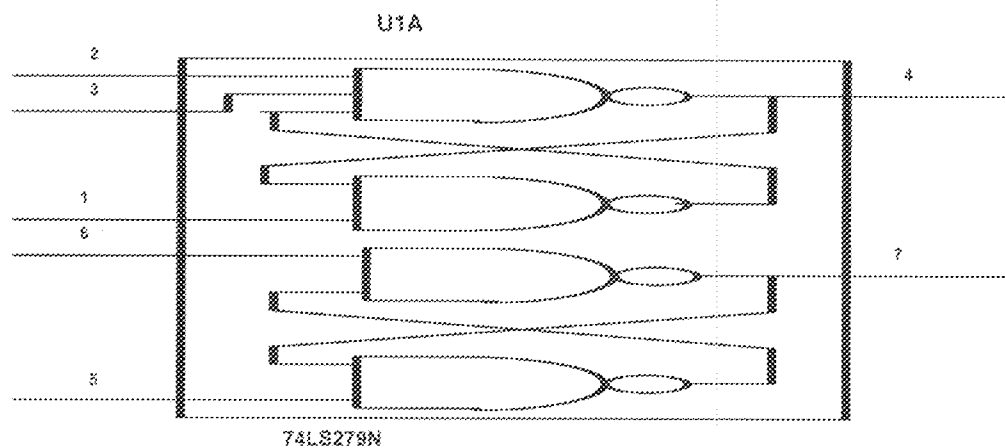
Fig.3.6 S-R Latch
