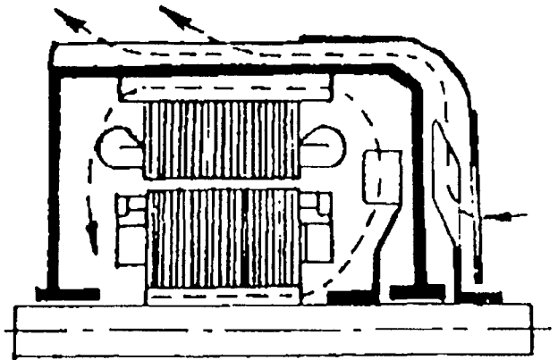
Fig 2 Internal fan circulator
