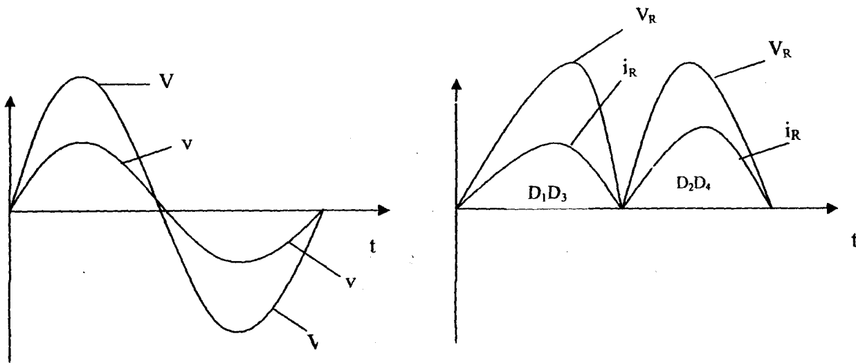
Fig. 3.4 (a) Sinusoidal input voltage
