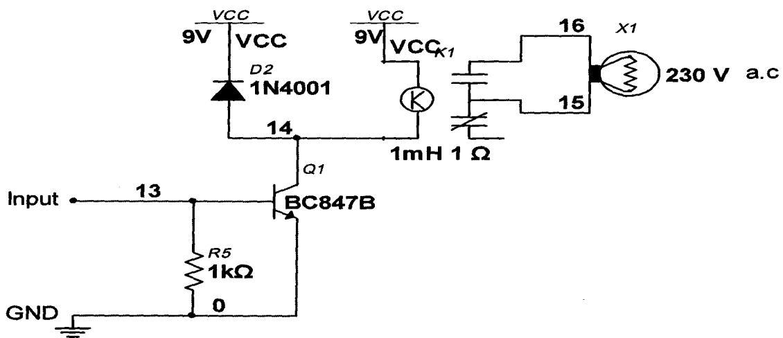
Fig: 3.9 Switching module
