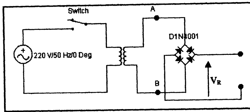
Fig. 3.7.2 Bridge rectifier circuit.
