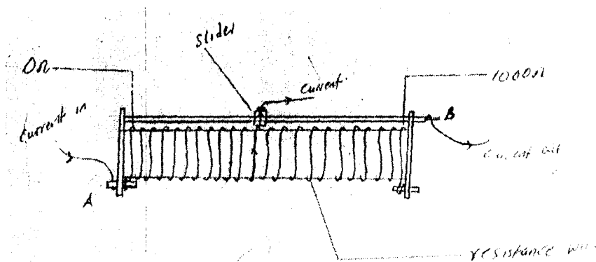
Fig. 3.0: Rheostat
