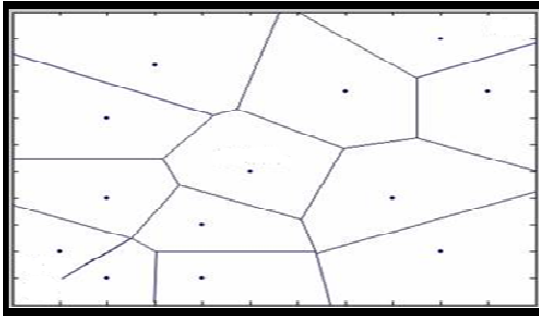
Fig 4. Voronoi polygon
