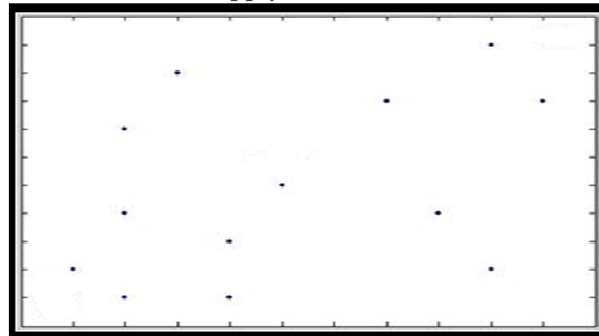
Fig 3. Voronoi point
